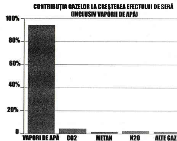
Figura 5. Acest grafic al gazelor cu efect de seră oferă o perspectivă de ansamblu asupra lăteriei legate de dioxidul de carbon. Dacă doriți să opriți efectul de seră, atunci interziceți norii și condensarea și, apropo, este necesar să avem în vedere că fără efectul de seră și fără dioxid de carbon (CO2) nu ar exista viața umană.
